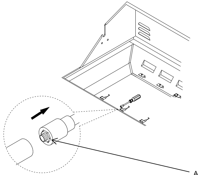
A. Main burner orifice
