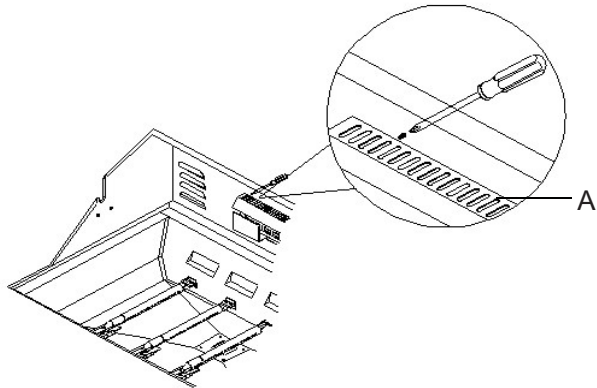
A. Wind Baffle
